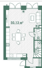
План 1 этажа
